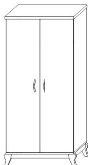
F8 Szafa 800/1950/600
