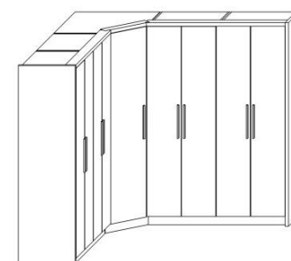
E19 Szafa 250 x 250 2572 x 2572 / 2136 / 600
