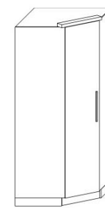
E12 Segment 90x90 900 / 2136 / 900
