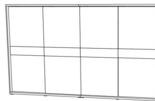
MD 05 Szafa przesuwana 4 drzwkowa 3200/2100/650 mm (S/W/G)
