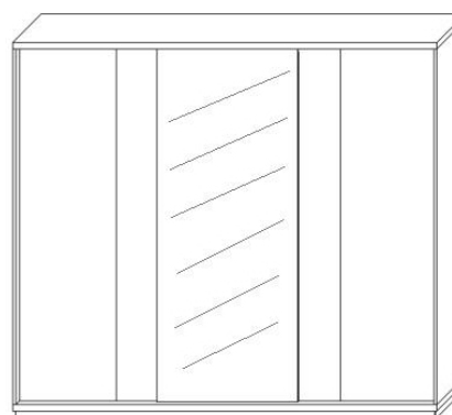
MS 8 Szafa przesuwana 3 drzwi – 2400/2122/650
